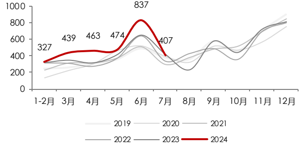
图表 2：24 年 7 月，电网基本建设投资完成额为 407 亿元，同减 2.9%
