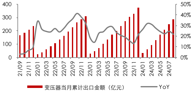
图表 3：24 年 1-8 月，中国变压器出口累计金额 285.9 亿元，同增 21.8%
