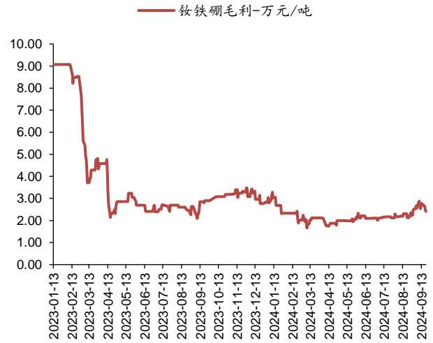
图 25：钕铁硼盈利变化（万元/吨）
