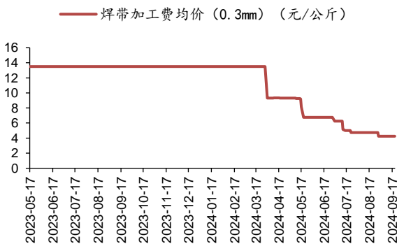
图 31：焊带加工费均价（0.3mm）走势(元/公斤)
