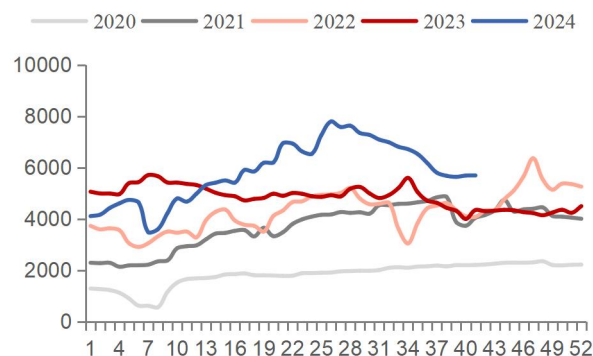
图表 27: 氢氧化锂周度产量 (吨)
