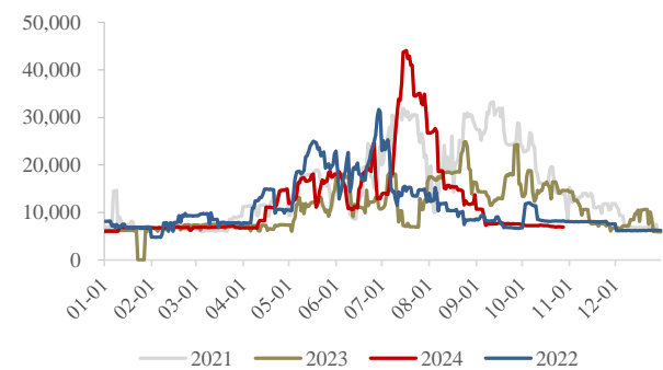
图6: 2021-2024 年三峡出库流量跟踪 (立方米/秒)
