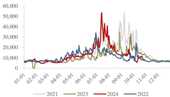
图5: 2021-2024 年三峡入库流量跟踪 (立方米/秒)
