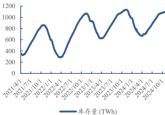
图18: 2021/4-2024/10 欧洲天然气库存量 (TWh)
