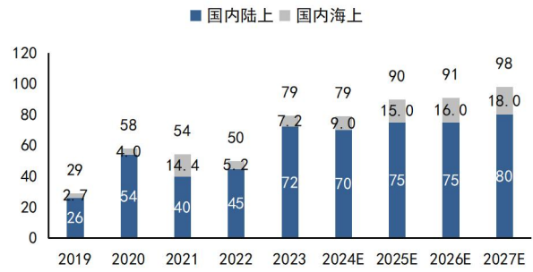
图14: 全国风电年度新增吊装容量走势（GW）
