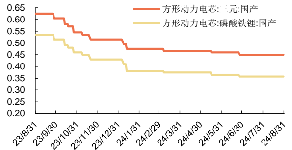
图14: 电池价格 (元/Wh)
